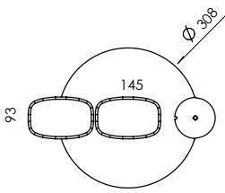
Moduł środkowy
